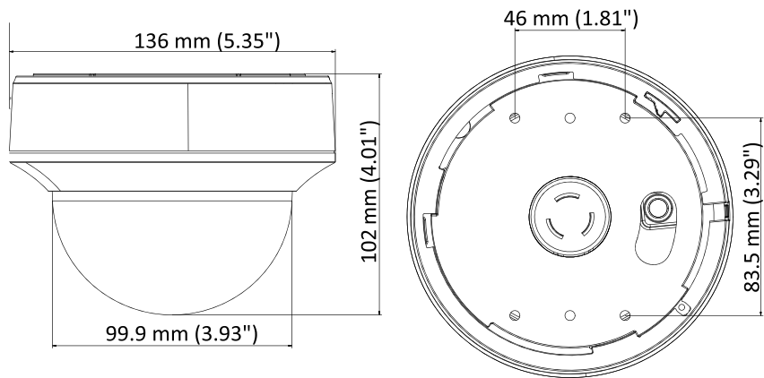
寸法図
