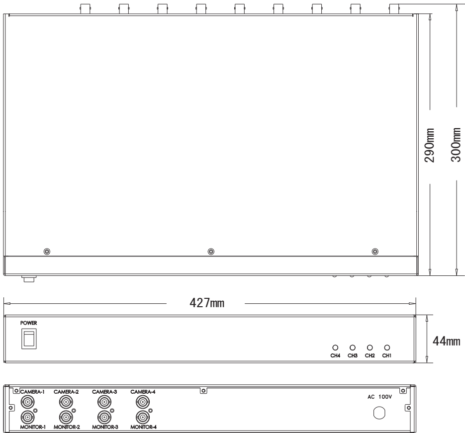
承認図
