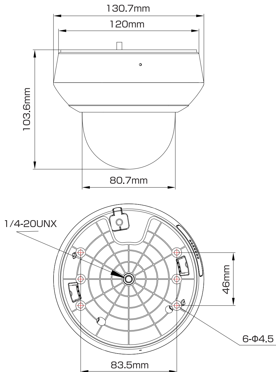
承認図
