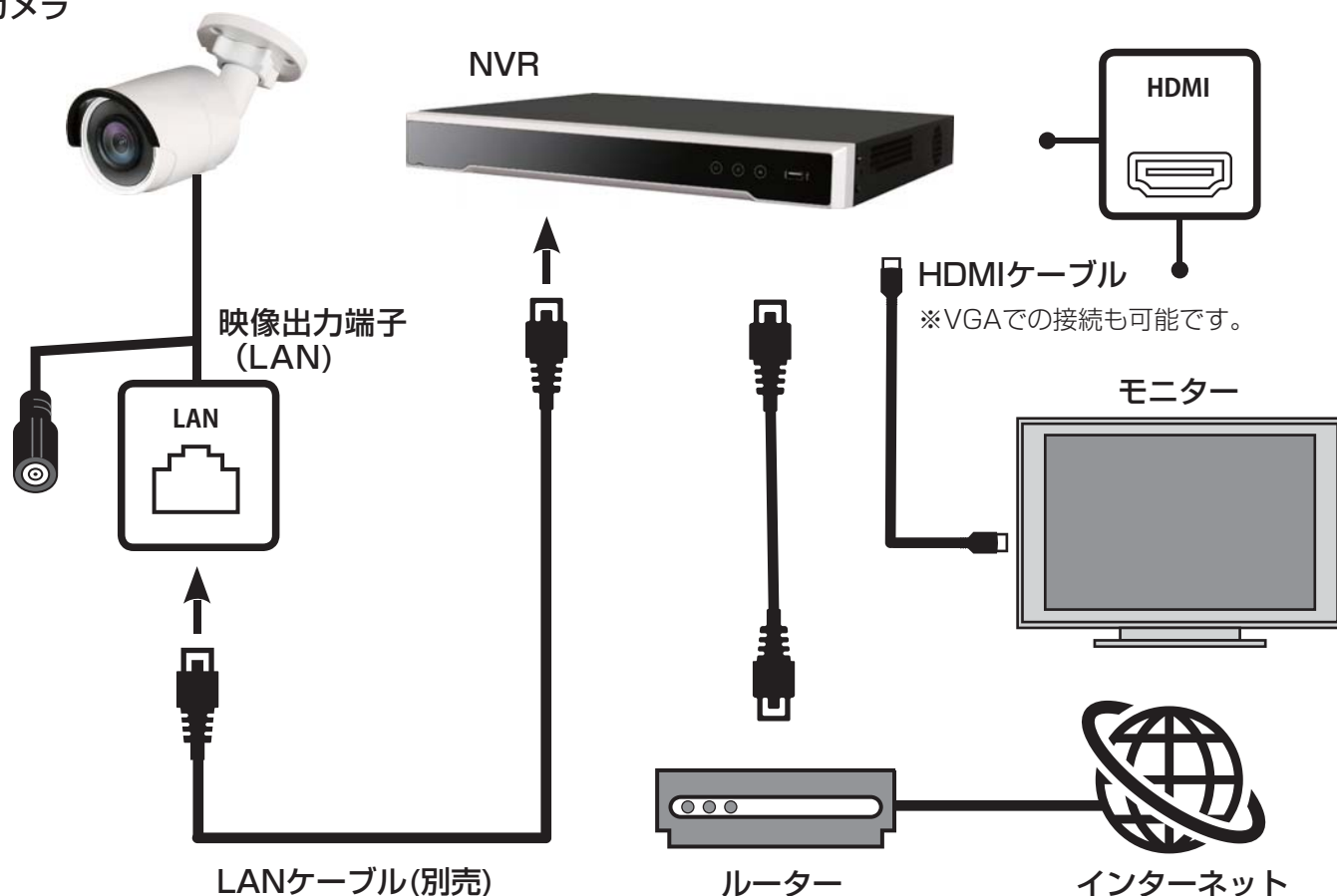
防犯カメラ
