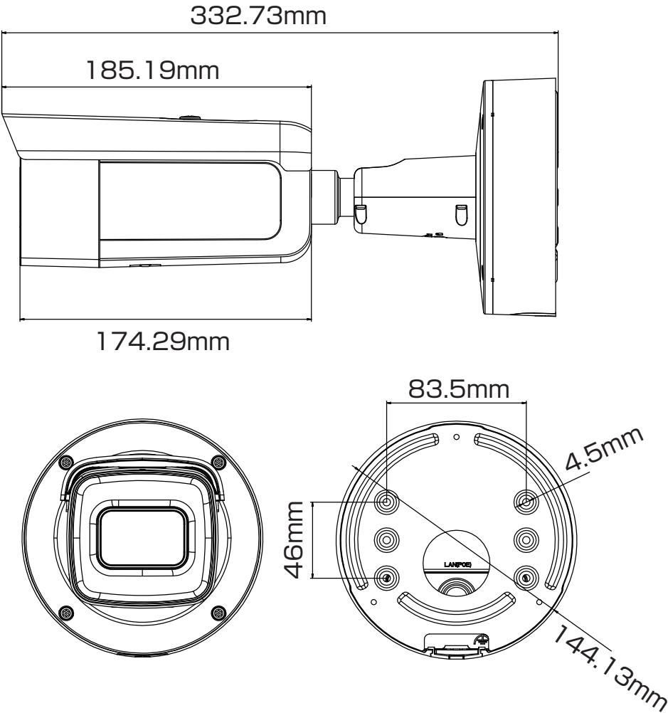
承認図
