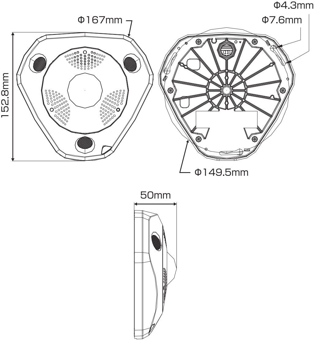
承認図
