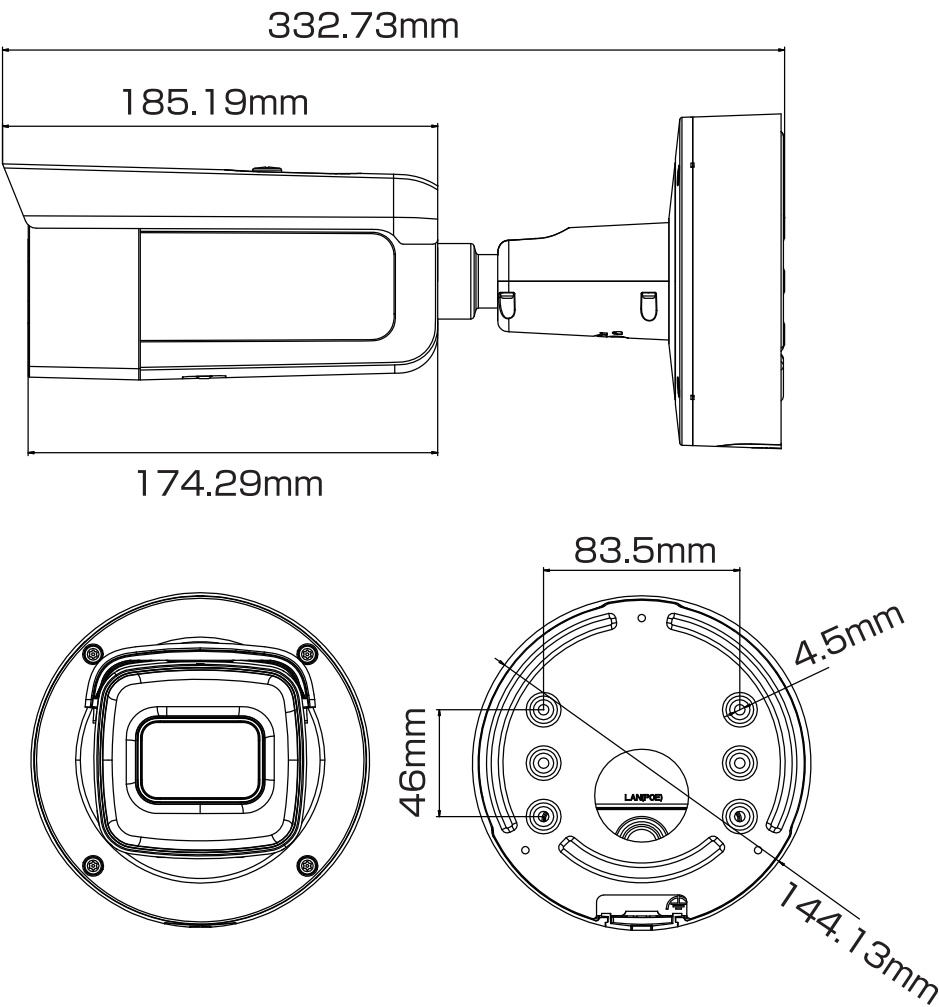
承認図
