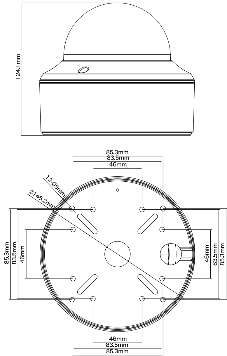
承認図
