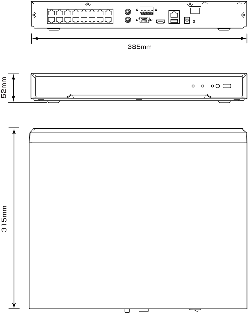
承認図
