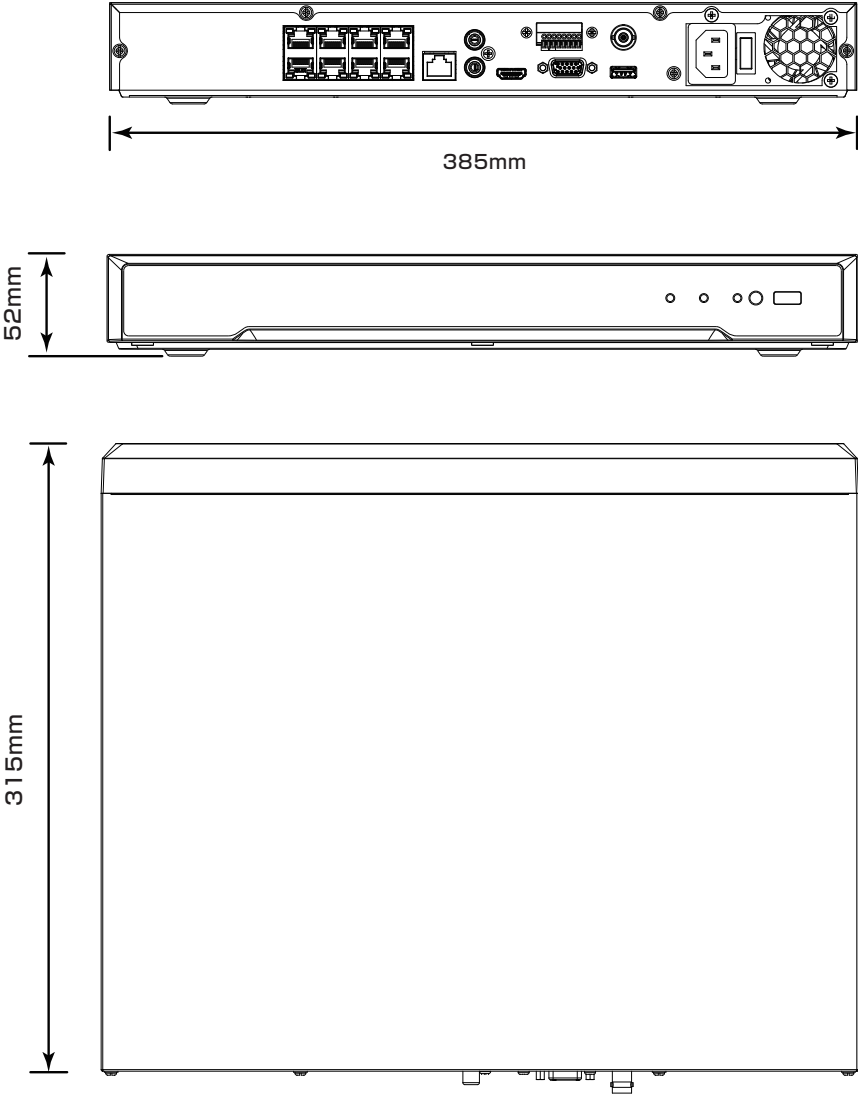
承認図
