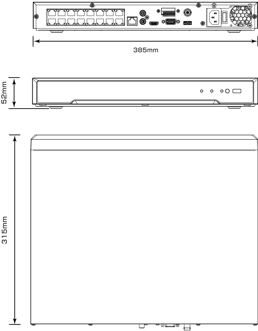
承認図
