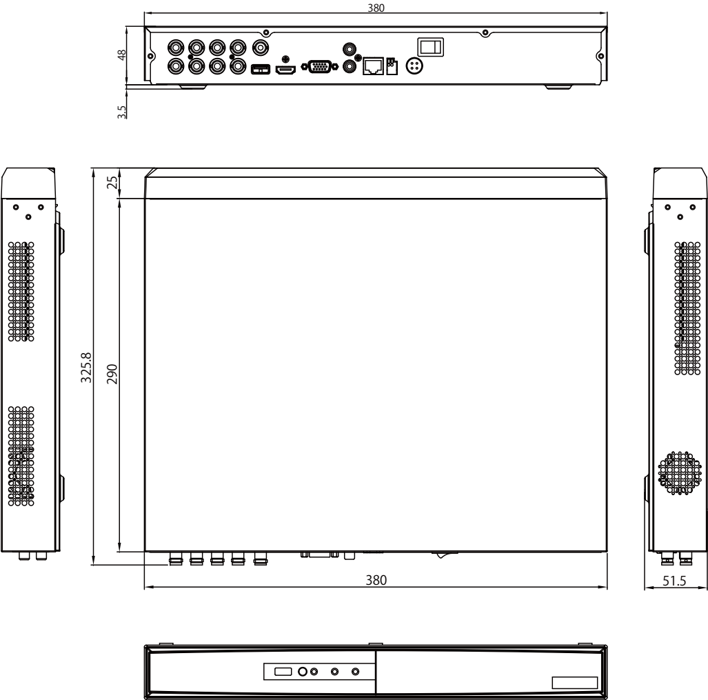
承認図
