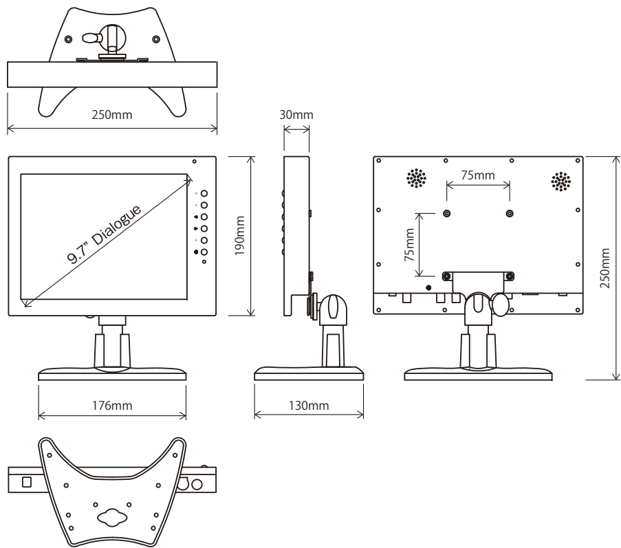
承認図
