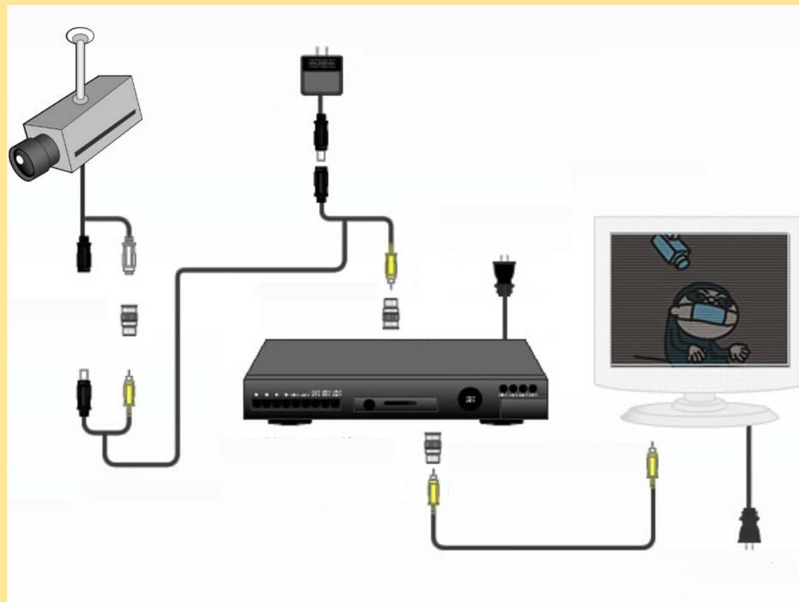
《カメラの配線例》
